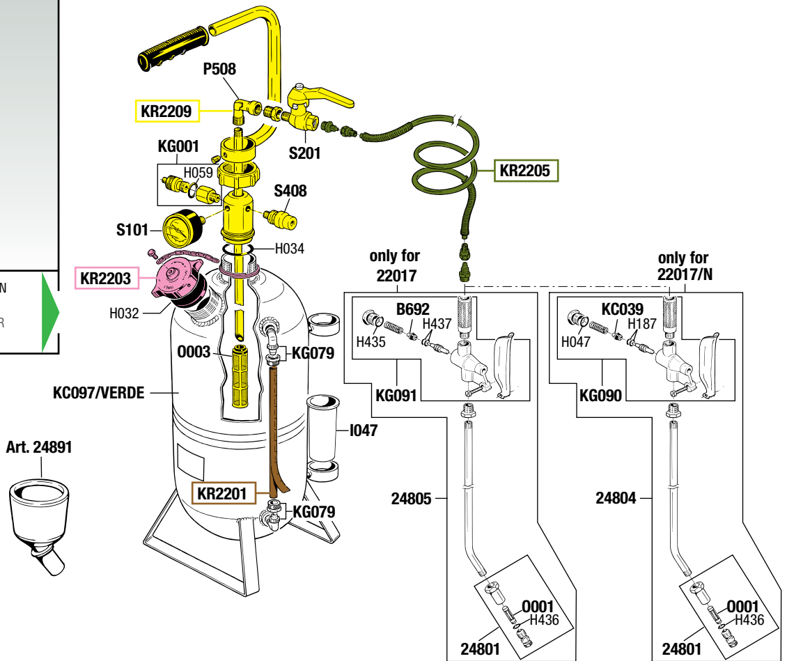
NEBULIZZATORE PORTATILE CON SERBATOIO DA 16 l PORTABLE PRESSURE SPRAYER WITH 16 l TANK
